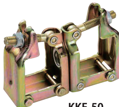
KKF-50 50 角角クランプ自在
