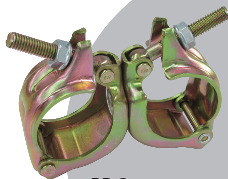
PP-3 Φ60.5×Φ60.5 クランプ自在 規格 /Φ60.5×Φ60.5 入数 /20個 単重 /760g
