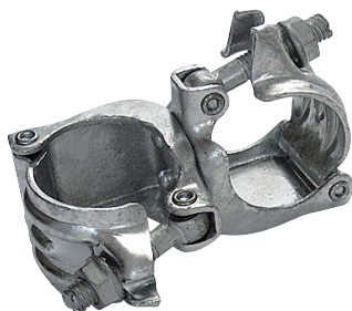
φ48.6クランプ直交 規格 / φ48.6×φ48.6 入数 / 30 個 単重 / 640g ※溶融亜鉛メッキ（ドブメッキ）仕様
