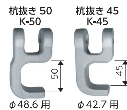
φ48.6 用
