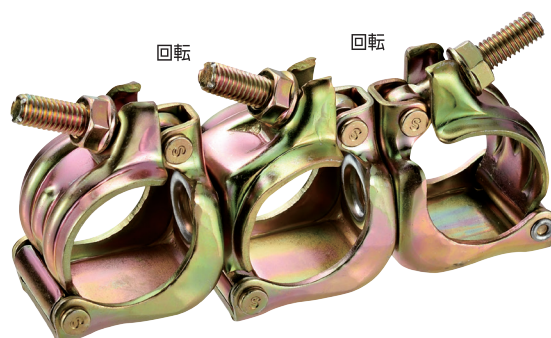
SFF-48 三連自在クランプ 規格 / \phi 48.6 \times \phi 48.6 \times \phi 48.6 入数 / 20 個 単重 / 1.05kg
