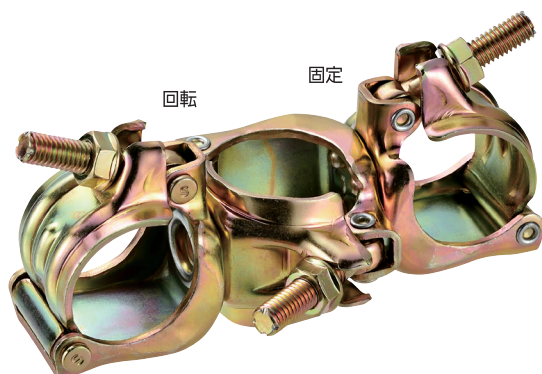
SSF-48 三連直交クランプ 規格 / \phi 48.6 \times \phi 48.6 \times \phi 48.6 入数 / 20 個 単重 / 1.05kg
