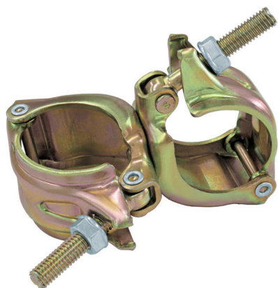
PP-1 \phi 60.5 \times \phi 60.5 クランプ直交 受注生産 規格 / \phi 60.5 \times \phi 60.5 入数 / 20 個 単重 / 760g
