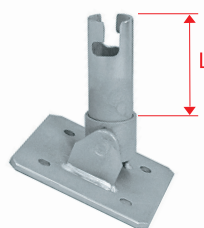
自在ベース
