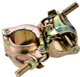
NCS-42 φ42.7クランプ直交 規格 / φ42.7×φ42.7 入数 / 30 個 単重 / 580g ※φ48.6×φ48.6 クランプ有り
