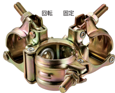
MAC-1 マルチクランプ直交 規格 / \phi 48.6 \times \phi 48.6 \times \phi 48.6 入数 / 10 個 単重 / 1.1kg
