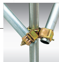
MAC-2 マルチクランプ自在 規格 / \phi 48.6 \times \phi 48.6 \times \phi 48.6 入数 / 10 個 単重 / 1.1kg
