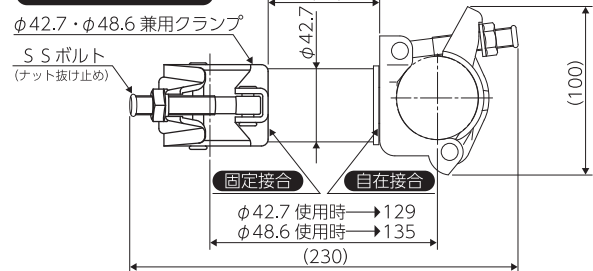
ツナギクランプ寸法図
