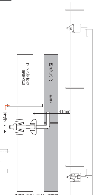
●養生クランプ Ne 使用図
