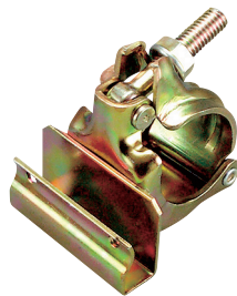
板止めクランプ平行 入数 / 40 個 単重 / 440g 金具部 / 厚さ 12mm 板用 止め穴 \phi 5 用 4ヶ所
