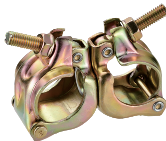
NCF-42 φ42.7クランプ自在 規格 / φ42.7×φ42.7 入数 / 30 個 単重 / 580g ※φ48.6×φ48.6 クランプ有り
