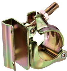
板止めクランプ直交 入数 / 40 個 単重 / 440g 金具部 / 厚さ 12mm 板用 止め穴 \phi 5 用 4ヶ所
