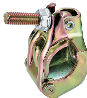
32-37単クランプ
