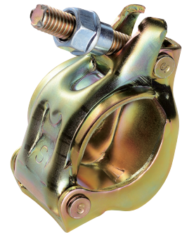
兼用単クランプ(ハイド) 規格 / φ48.6・φ42.7 兼用 スリーブナット仕様
