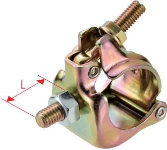
ボルト付単クランプ 規格 / φ48.6 1/2 ボルト L=28mm その他各種単クランプや、 その他のボルトに変更可能
