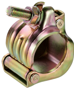
φ42.7単クランプ 規格 / φ42.7
