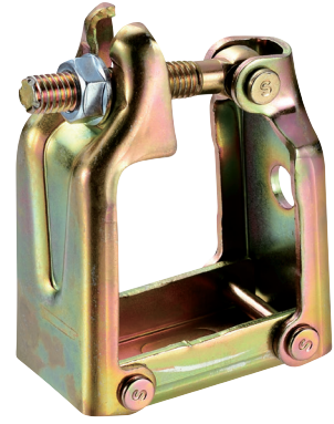
60角単クランプ 規格 /□60
