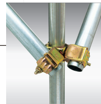
MAC-2 マルチクランプ自在 規格 / \phi 48.6 \times \phi 48.6 \times \phi 48.6 入数 / 10個 単重 / 1.1kg
