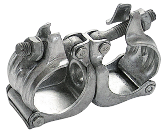
φ48.6クランプ自在 規格 / φ48.6×φ48.6 入数 / 30個 単重 / 640g ※溶融亜鉛メッキ (ドブメッキ) 仕様
