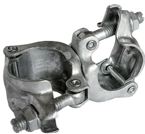
φ42.7クランプ直交 規格 / φ42.7×φ42.7 入数 / 30個 単重 / 620g ※溶融亜鉛メッキ (ドブメッキ) 仕様
